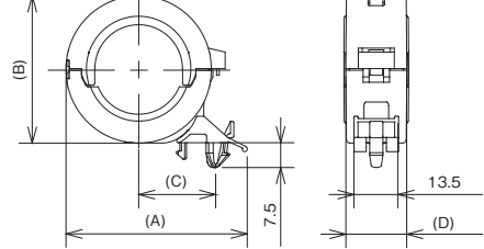
形状 / Profile②
