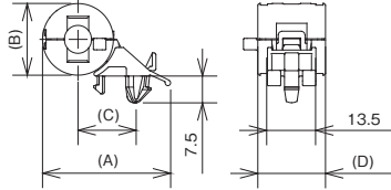
形状 / Profile①
