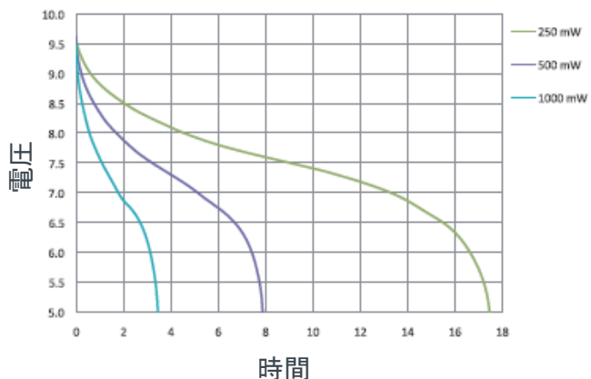
定電力放電
