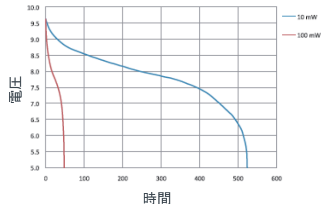
定電力放電
