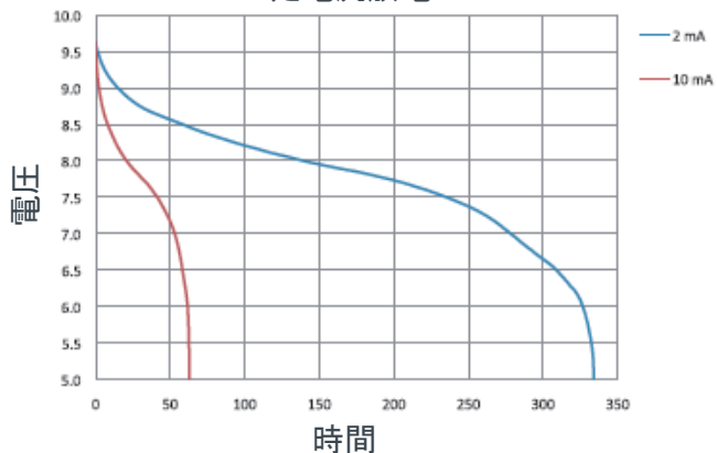
定電流放電
