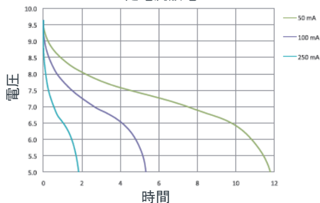
定電流放電
