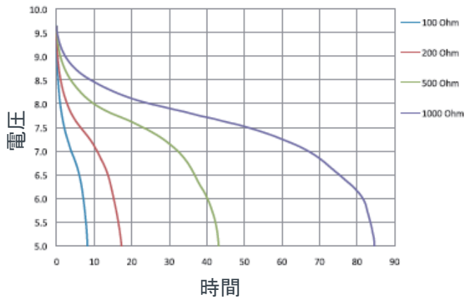
定抵抗放電
