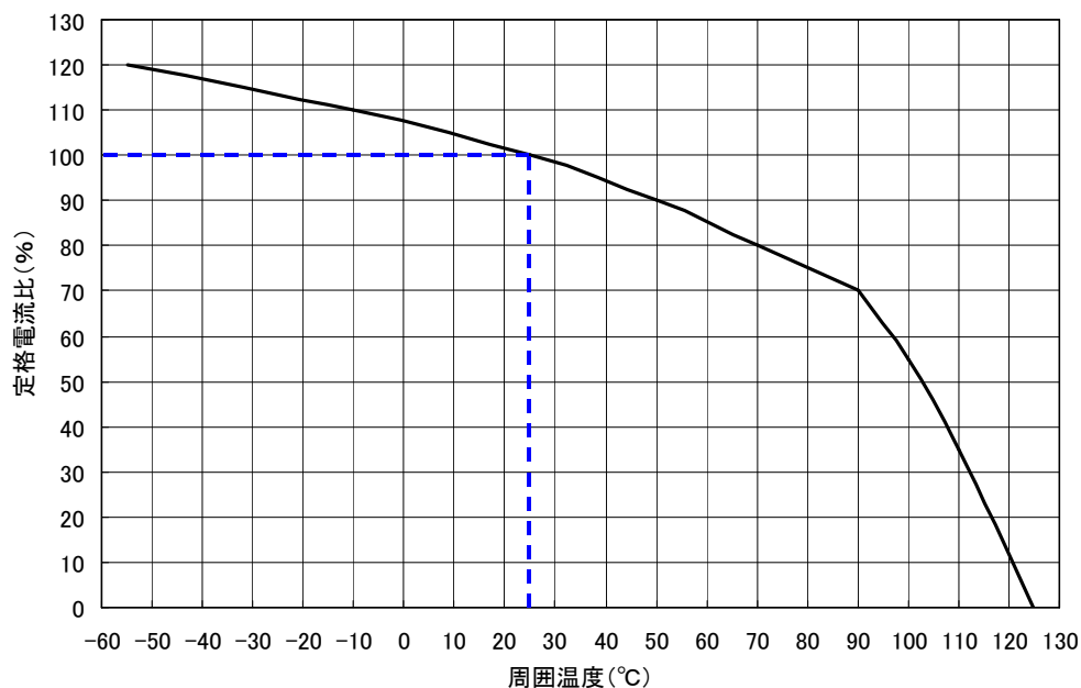
デレージング曲線
