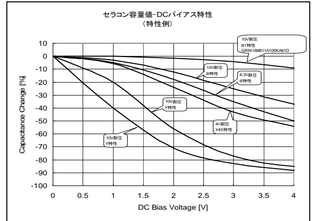
Figure 93. 容量-バイアス特性
