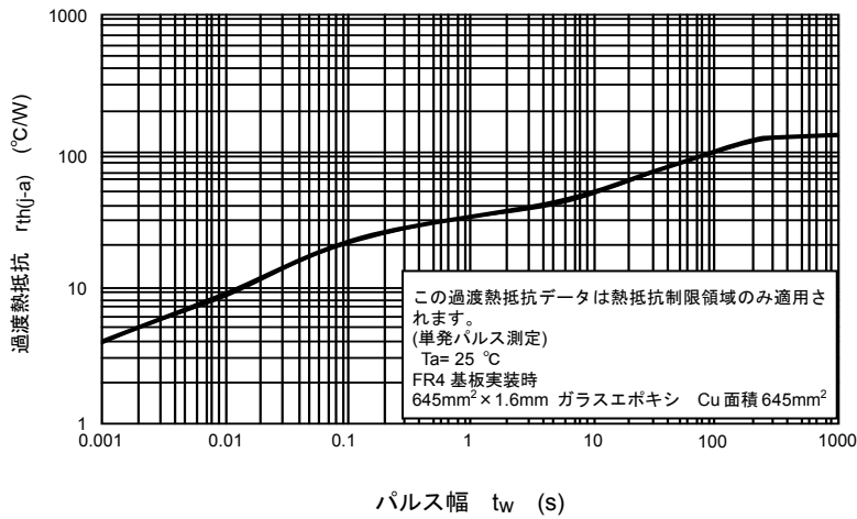
過渡熱抵抗 r_{th-tw}
