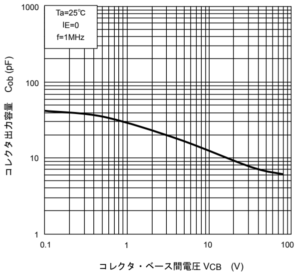
C_{ob} - V_{CB}
