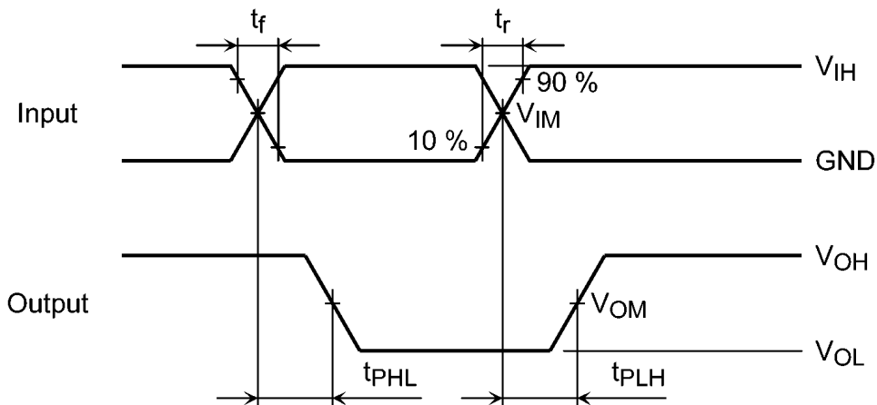
図 11.8.1 t_{PLH} , t_{PHL}
