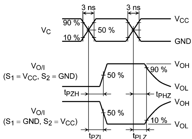
図 1 t_{PLZ} , t_{PHZ} , t_{PZL} , t_{PZH}
