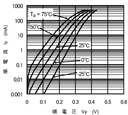
図 9.1 I_F - V_F
