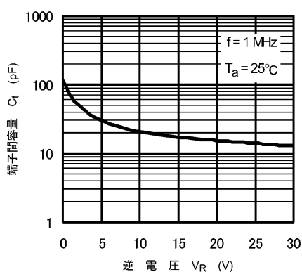
図 9.3 C_t - V_R
