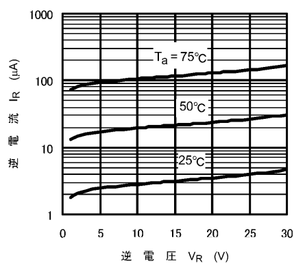
図 9.2 I_R - V_R
