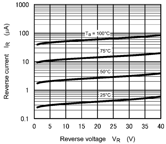
図 9.2 I_R - V_R
