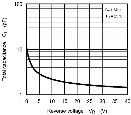
図 9.3 C_t - V_R
