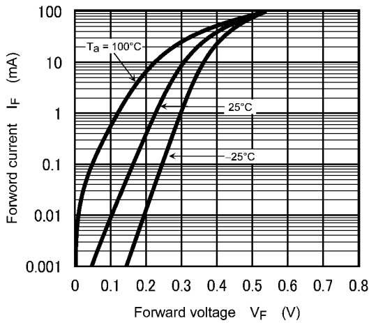
図 9.1 I_F - V_F
