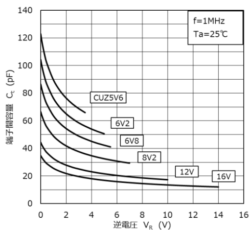
C_t - V_R (1)
