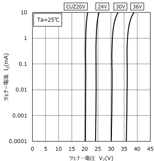
I_Z - V_Z (2)
