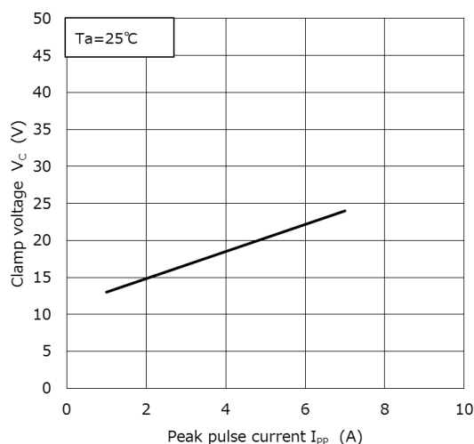
V_C - I_{PP} (注 2)
