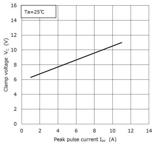
V_C - I_{PP} (注 2)
