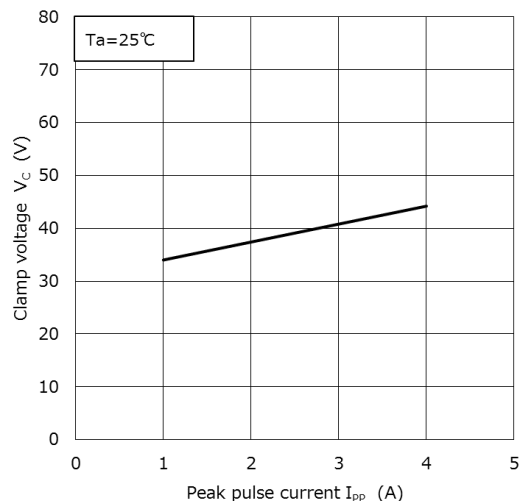
V_C - I_{PP} (注 2)
