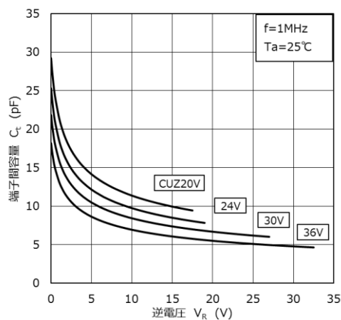
C_t - V_R (2)
