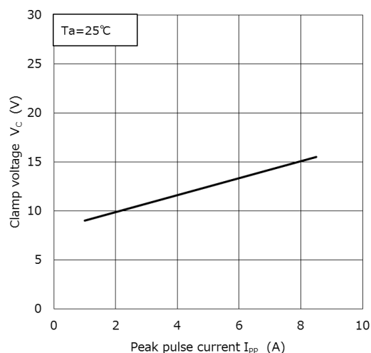
V_C - I_{PP} (注 2)
