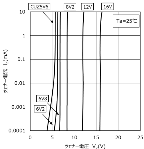
I_Z - V_Z (1)
