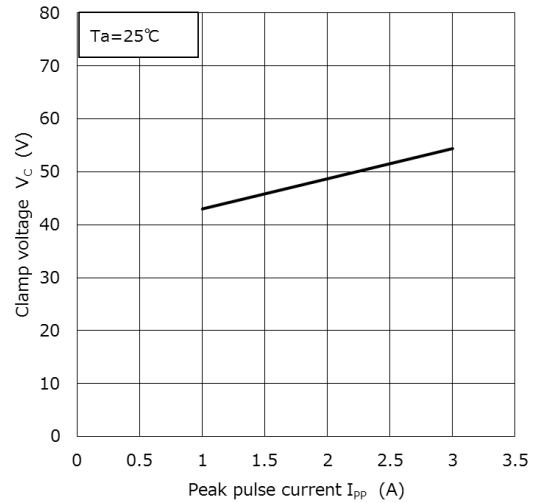
V_C - I_{PP} (注 2)
