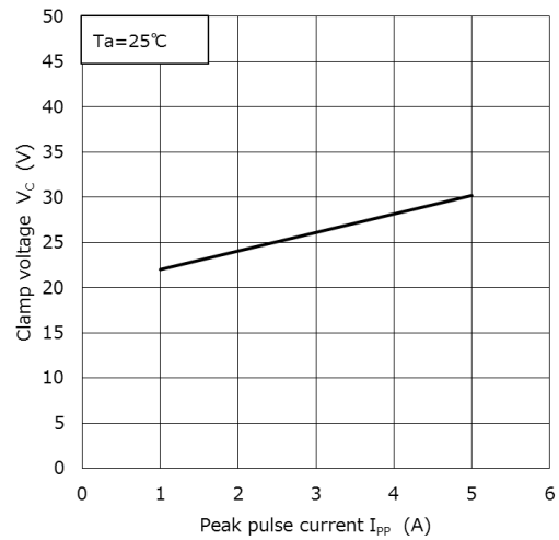
V_C - I_{PP} (注 2)
