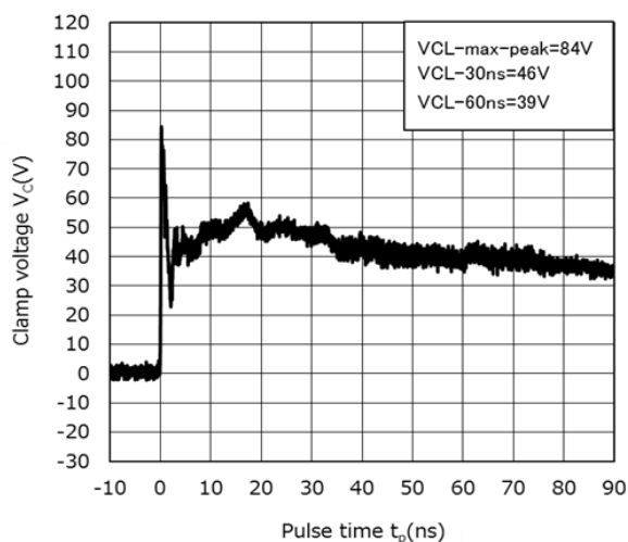
クランプ波形 +8 kV(注 3)
