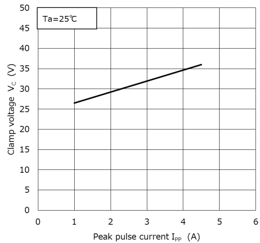
V_C - I_{PP} (注 2)
