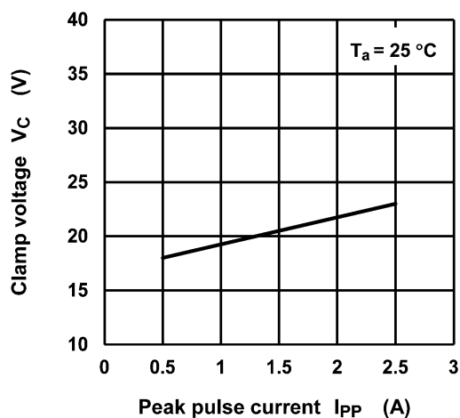
図 9.1 V_C - I_{PP}
