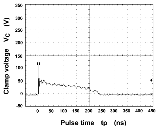
図 10.1 +8 kV
