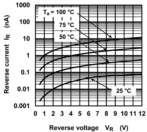
図 8.2 I_R - V_R
