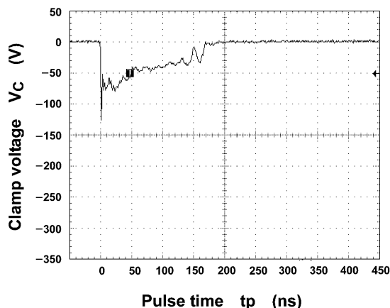
図 10.2 -8 kV
