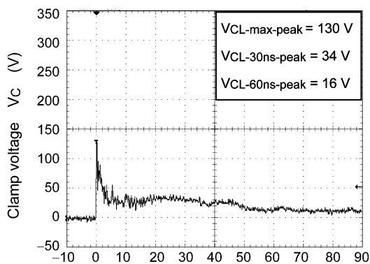
図 6.1.3 +15 kV
