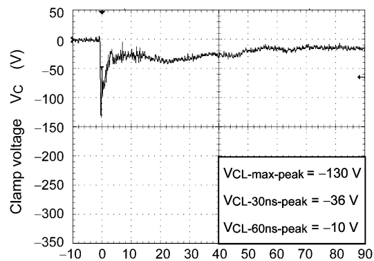
図 6.1.4 -15 kV
