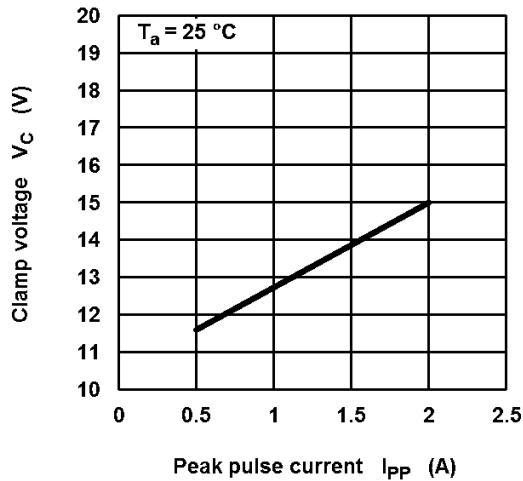
図 8.1 V_C - I_{PP}
