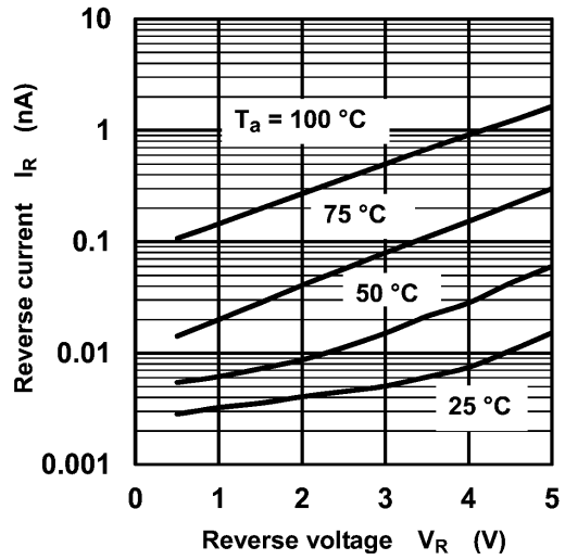
図 7.2 I_R - V_R
