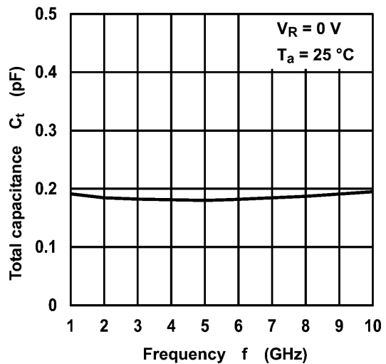
図 7.4 C_t - f
