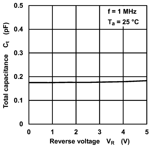
図 7.3 C_t - V_R
