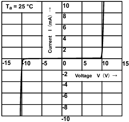
図 7.1 I - V
