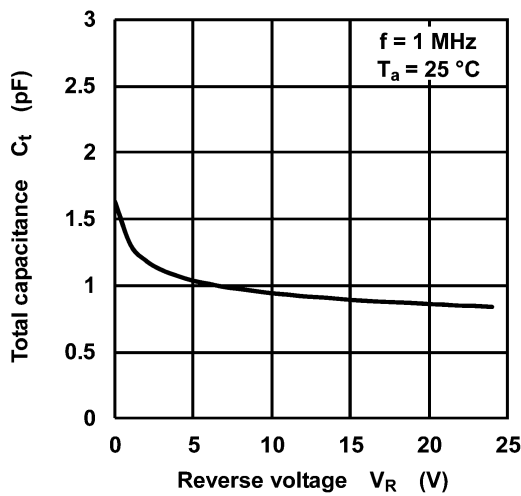
図 8.4 C_t - V_R
