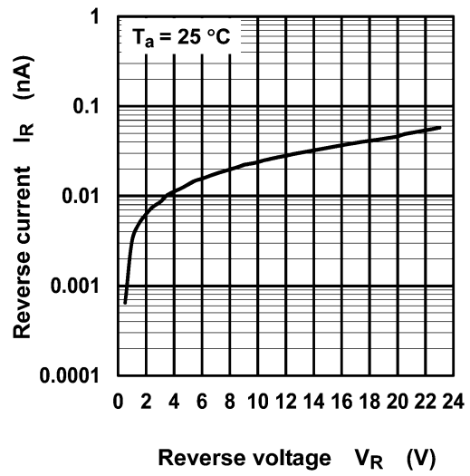
図 8.2 I_R - V_R
