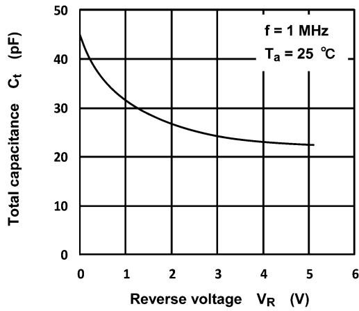
図 8.3 C_t - V_R
