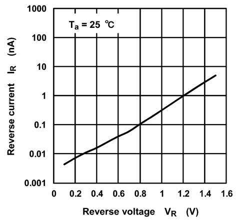
図 8.2 I_R - V_R
