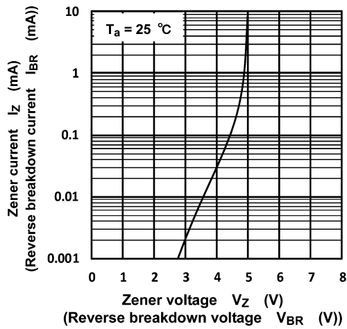
図 8.1 I_Z - V_Z (I_{BR} - V_{BR})
