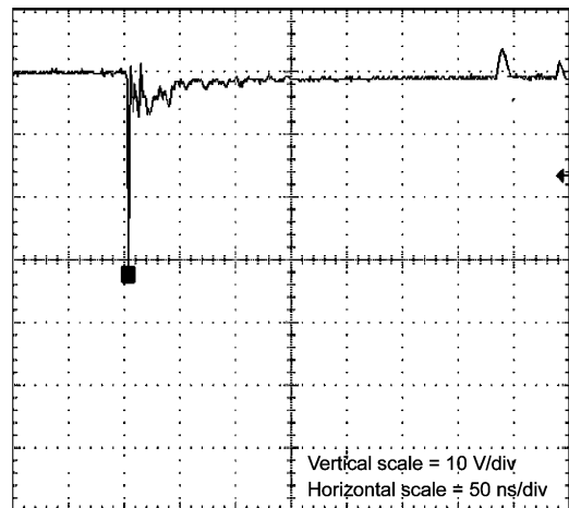
図 10.2 -8 kV
