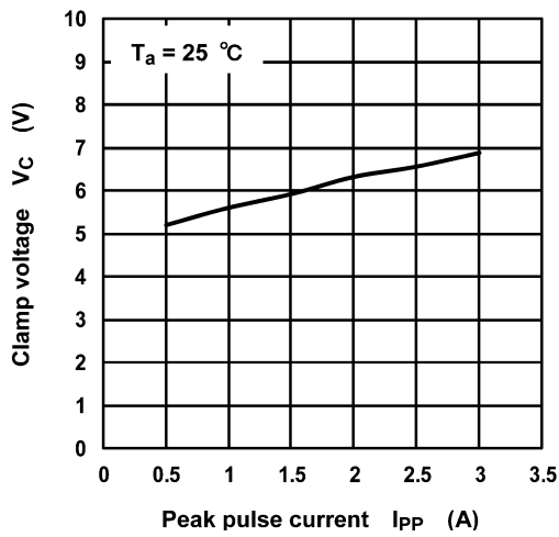
図 9.1 V_C - I_{PP}
