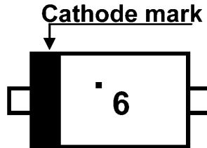
図 6.1 現品表示
