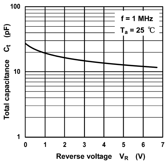
図 8.3 C_t - V_R
