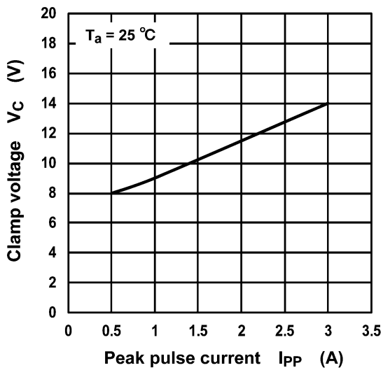
図 9.1 V_C - I_{PP}
