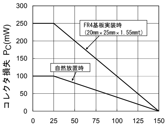
P_C - T_a
