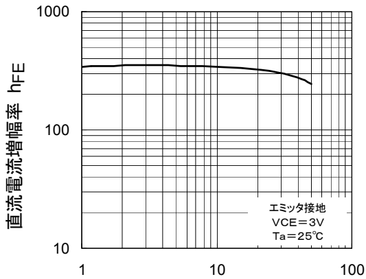
h_{FE}-I_C
