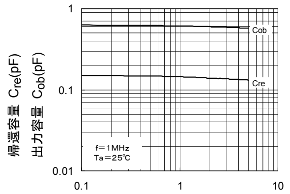
C_{re}, C_{ob}-V_{CB}
