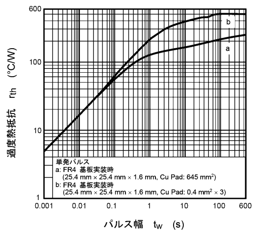
図 8.12 r_{th} - t_w
