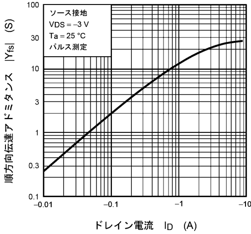
図 8.7 |Y_{fs}| - I_D
