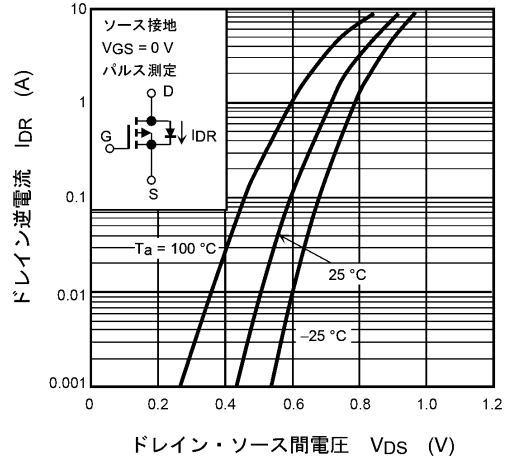
図 8.8 I_{DR} - V_{DS}
