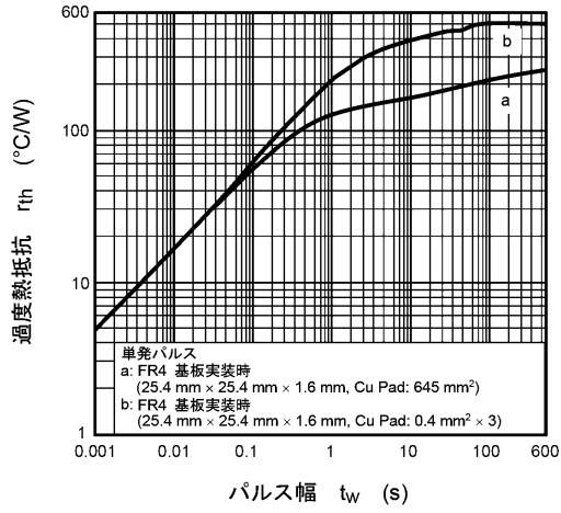
図 8.13 r_{th} - t_w
