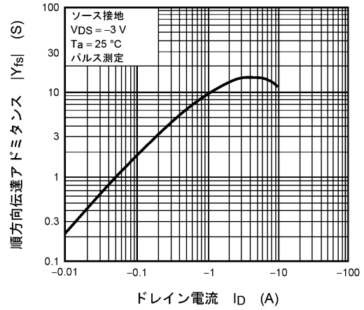
図 8.8 |Y_{fs}| - I_D
