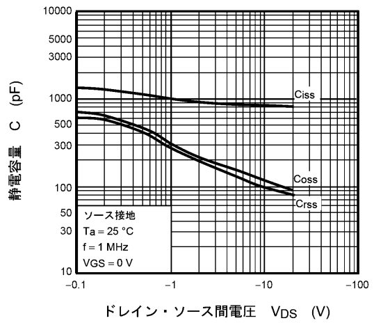
図 8.10 C - V_{DS}
