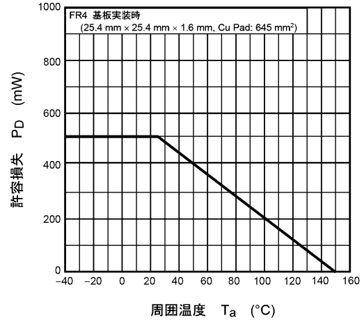
図 8.14 P_D - T_a
