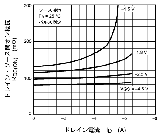
図 7.4 R_{DS(ON)} - I_D
