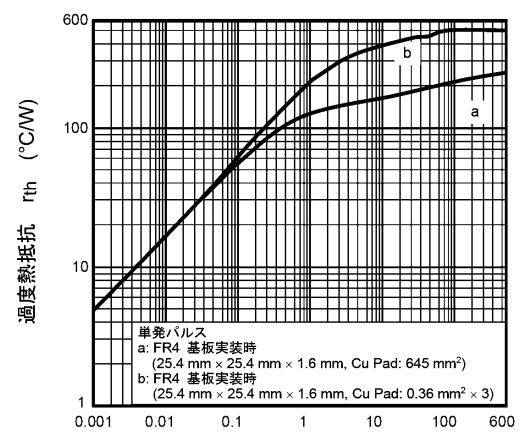
パルス幅 t_w (s) 図 7.12 r_{th} - t_w
