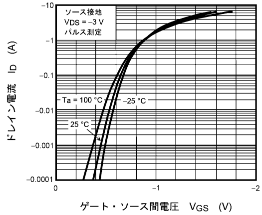
図 7.2 I_D - V_{GS}
