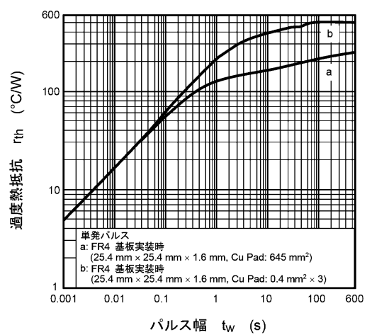
図 8.12 r_{th} - t_w
