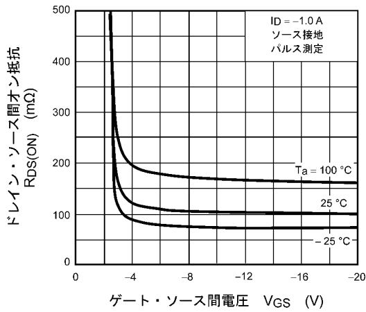
図 8.3 R_{DS(ON)} - V_{GS}
