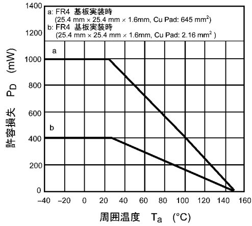
図 8.13 P_D - T_a
