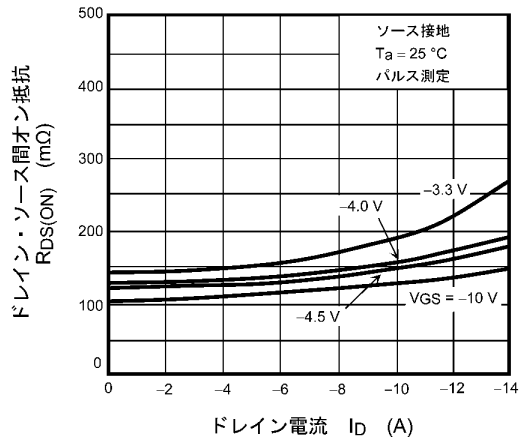
図 8.4 R_{DS(ON)} - I_D
