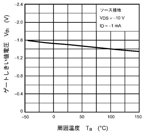
図 8.6 V_{th} - T_a
