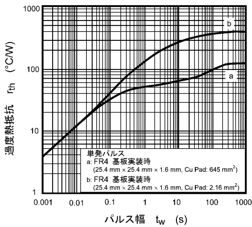
図 8.11 r_{th} - t_w
