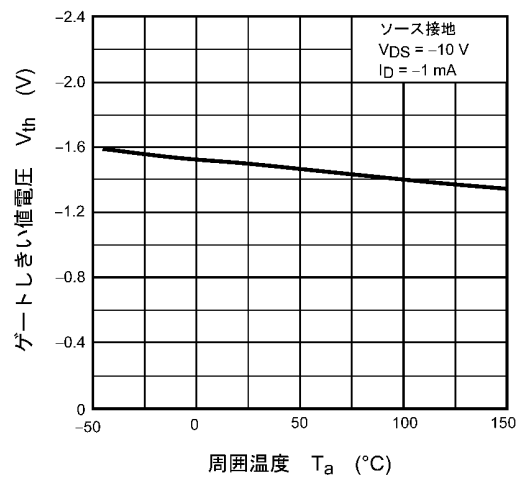
図 8.6 V_{th} - T_a
