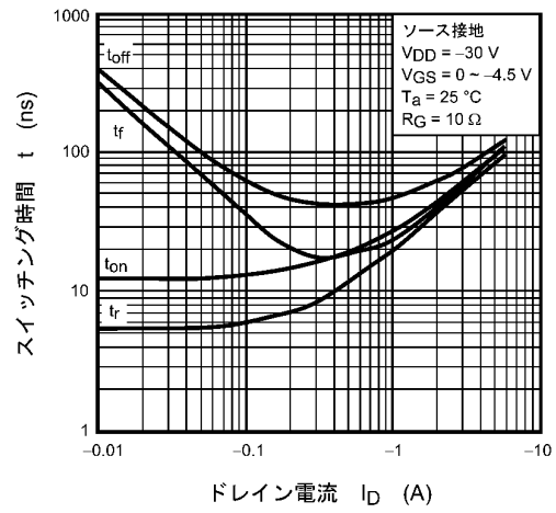
図 8.10 t - I_D
