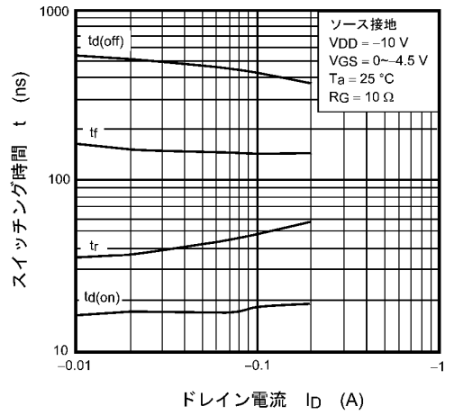
図 8.10 t - I_D
