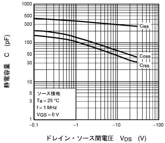
図 8.10 C - V_{DS}
