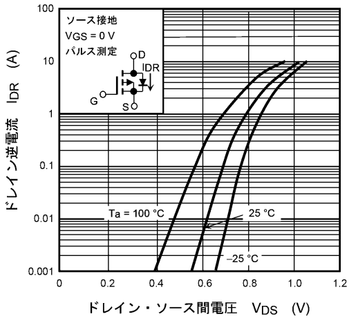
図 8.9 I_{DR} - V_{DS}
