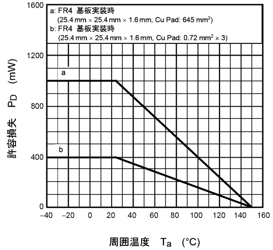
図 8.14 P_D - T_a
