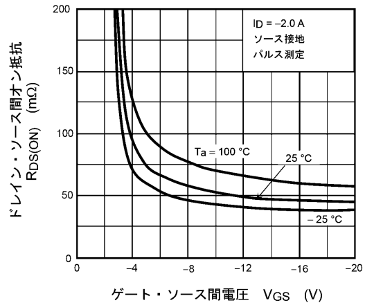
図 8.4 R_{DS(ON)} - V_{GS}
