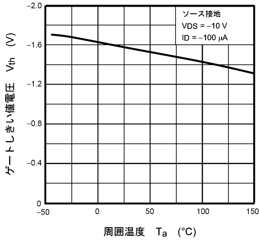
図 8.7 V_{th} - T_a
