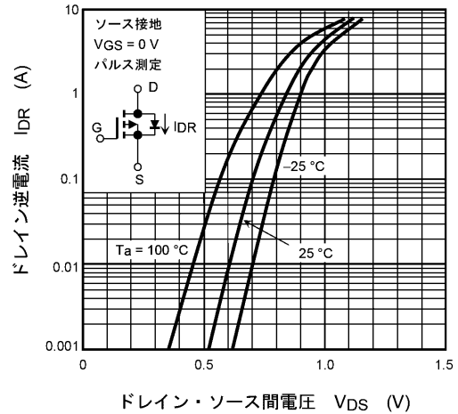
図 8.8 I_{DR} - V_{DS}
