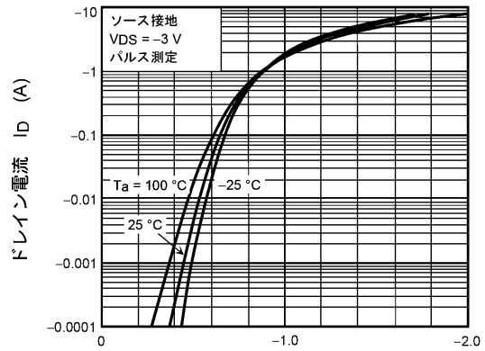
ゲート・ソース間電圧 V_{GS} (V)
