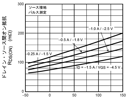
周囲温度 T_a (°C)
