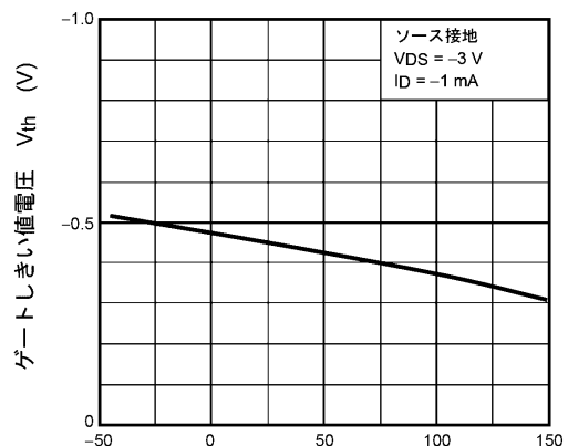
周囲温度 T_a (°C)
