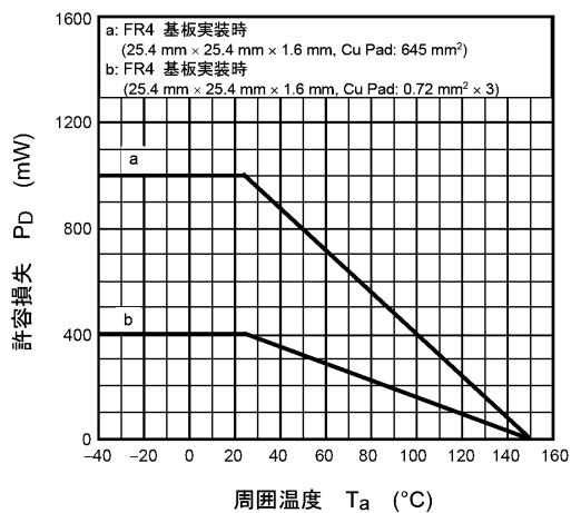
図 8.13 P_D - T_a
