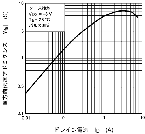
図 8.7 |Y_{fs}| - I_D
