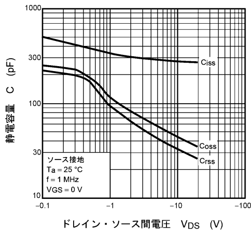
図 8.9 C - V_{DS}
