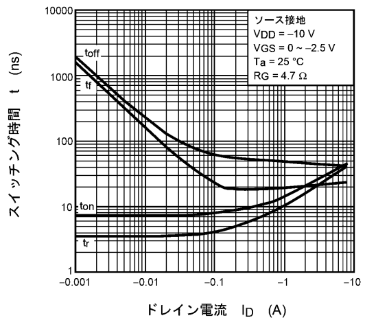
図 8.10 t - I_D
