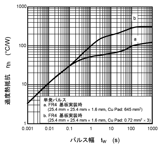
図 8.12 r_{th} - t_w
