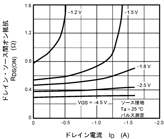
図 7.5 R_{DS(ON)} - I_D
