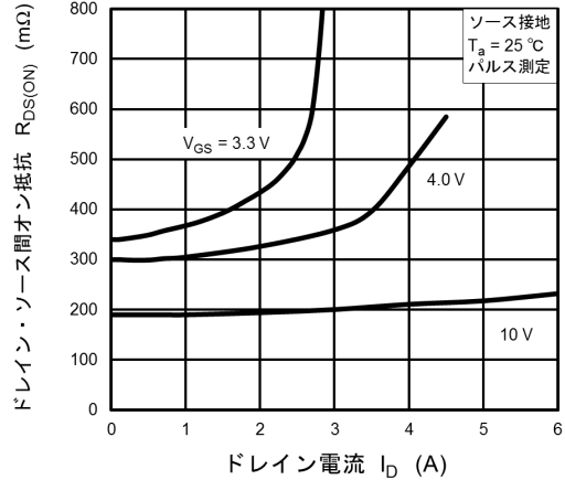
図 7.6 R_{DS(ON)} - I_D
