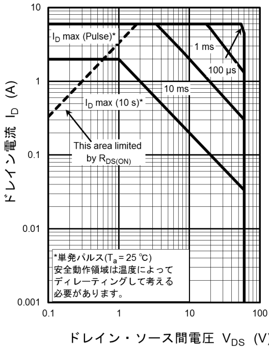
図 7.15 安全動作領域
