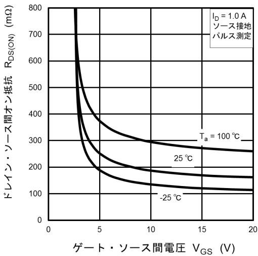
図 7.5 R_{DS(ON)} - V_{GS}
