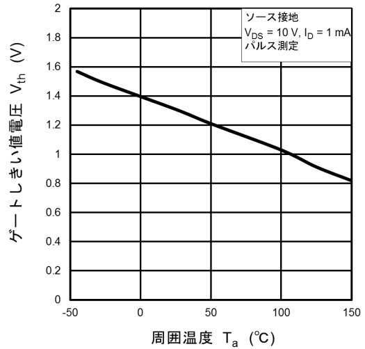
図 7.8 V_{th} - T_a
