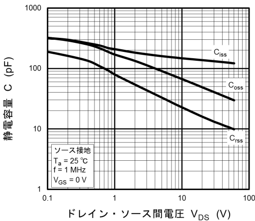
図 7.11 C - V_{DS}
