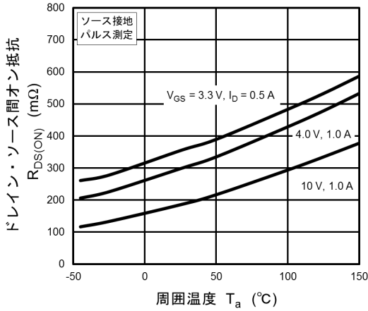
図 7.7 R_{DS(ON)} - T_a
