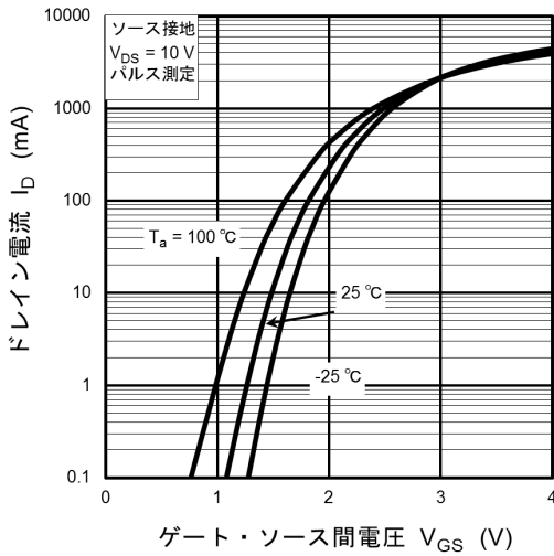
図 7.3 I_D - V_{GS}
