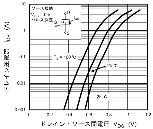
図 7.10 I_{DR} - V_{DS}
