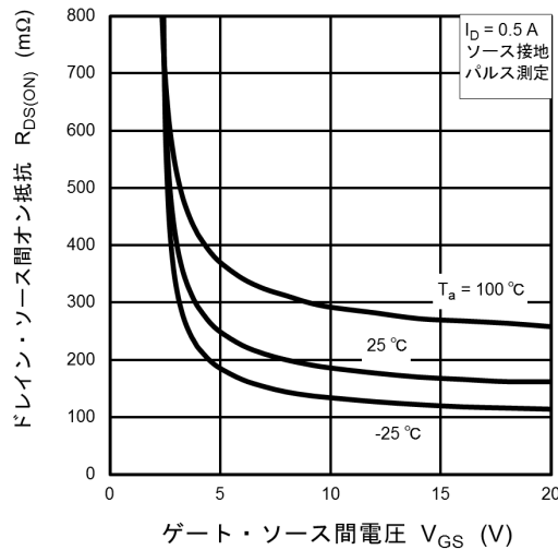
図 7.4 R_{DS(ON)} - V_{GS}
