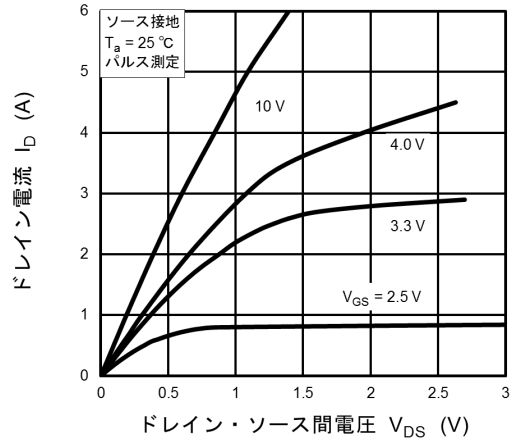
図 7.2 I_D - V_{DS}
