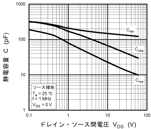
図 7.11 C - V_{DS}
