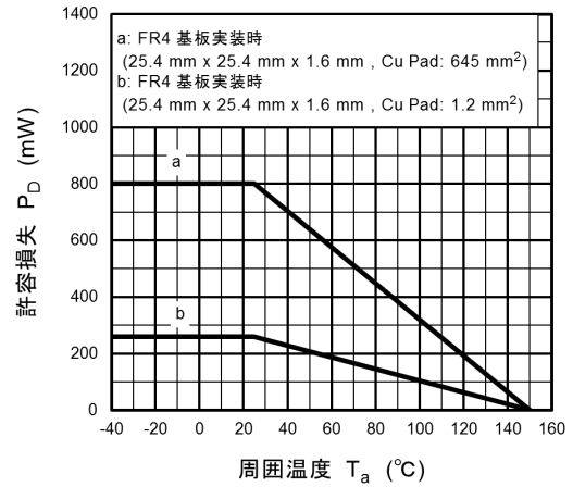
図 7.14 P_D - T_a
