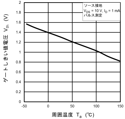
図 7.8 V_{th} - T_a
