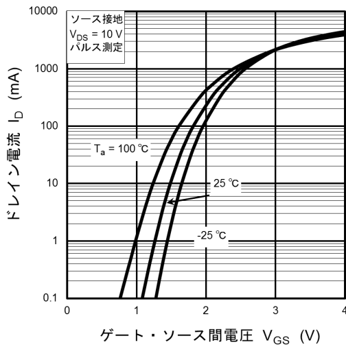
図 7.3 I_D - V_{GS}
