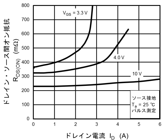
図 7.6 R_{DS(ON)} - I_D
