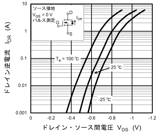
図 7.10 I_{DR} - V_{DS}
