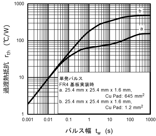
図 7.13 r_{th} - t_w
