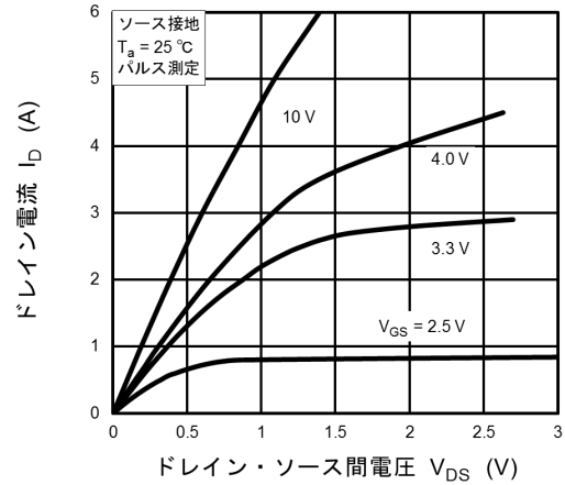
図 7.2 I_D - V_{DS}
