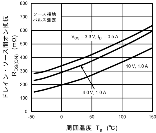
図 7.7 R_{DS(ON)} - T_a
