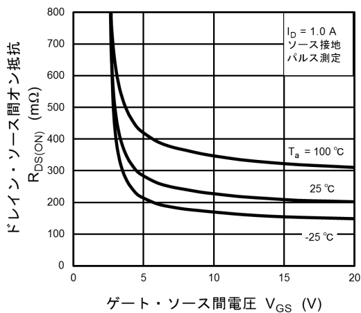
図 7.5 R_{DS(ON)} - V_{GS}
