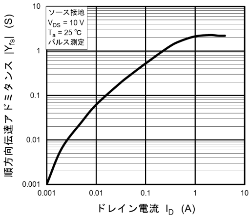
図 7.9 |Y_{fs}| - I_D
