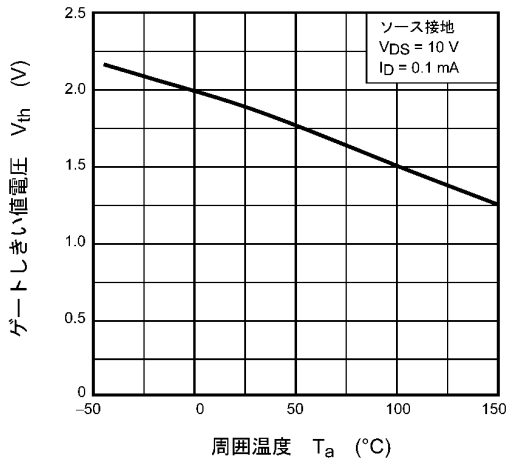
図 7.7 V_{th} - T_a
