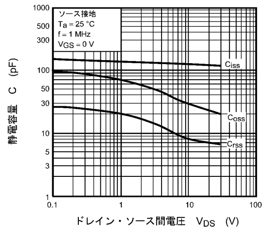
図 7.10 C - V_{DS}
