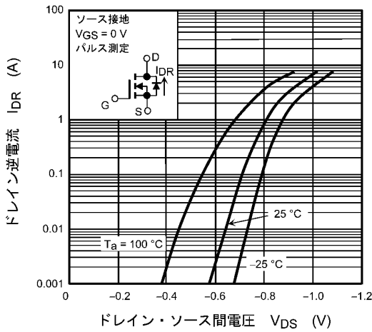
図 7.9 I_{DR} - V_{DS}
