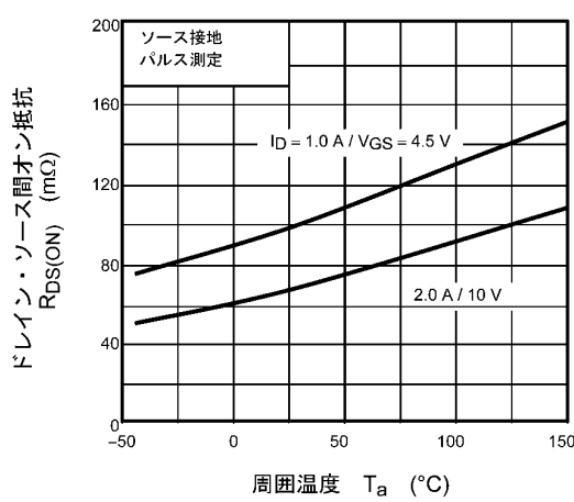
図 7.6 R_{DS(ON)} - T_a
