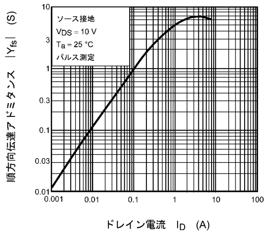
図 7.8 |Y_{fs}| - I_D
