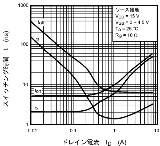
図 7.11 t - I_D
