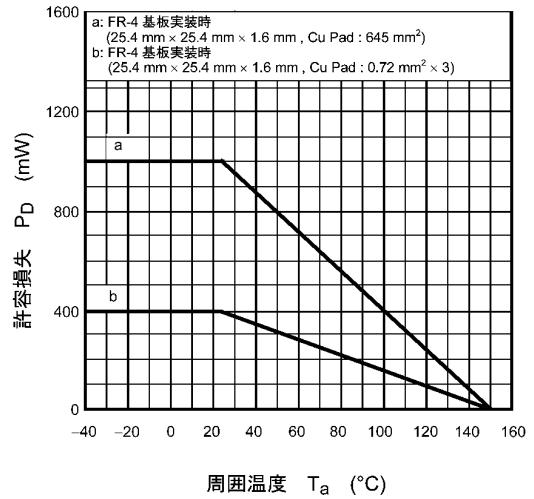
図 7.14 P_D - T_a
