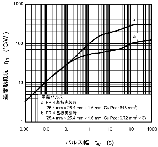
図 7.13 r_{th} - t_w
