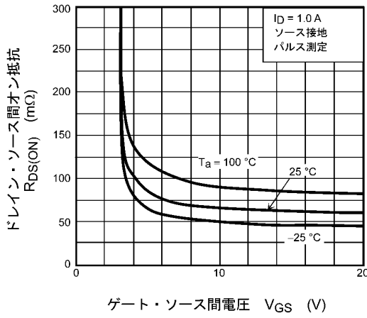
図 7.3 R_{DS(ON)} - V_{GS}
