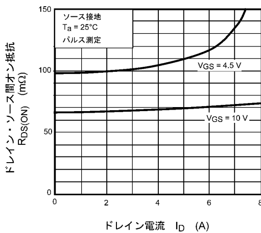
図 7.5 R_{DS(ON)} - I_D
