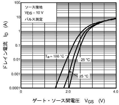
図 7.2 I_D - V_{GS}
