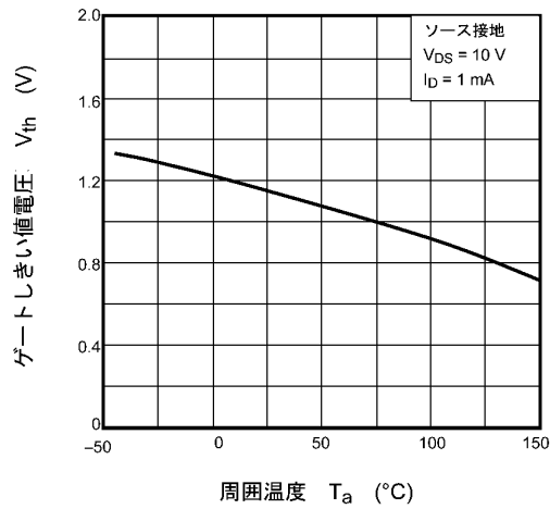
図 7.6 V_{th} - T_a
