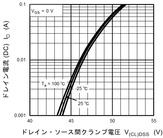
図 7.15 I_D - V_{(CL)DSS}
