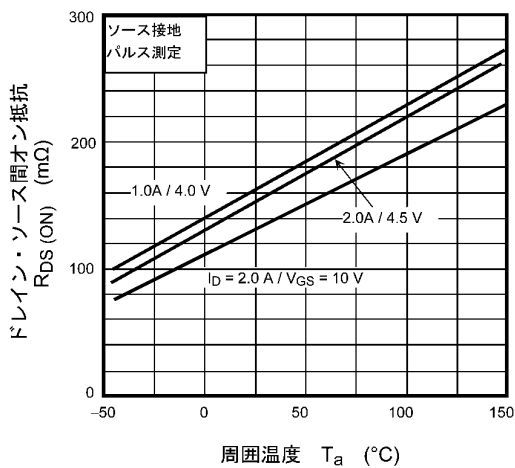
図 7.5 R_{DS(ON)} - T_a
