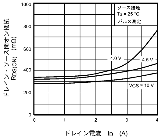
図 7.4 R_{DS(ON)} - I_D
