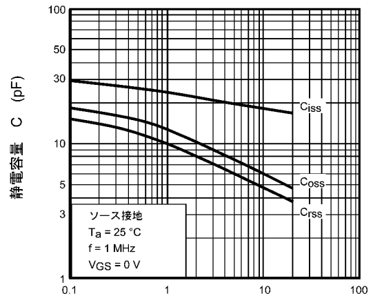
図 7.10 C - V_{DS}
