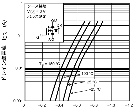
図 7.9 I_{DR} - V_{DS}
