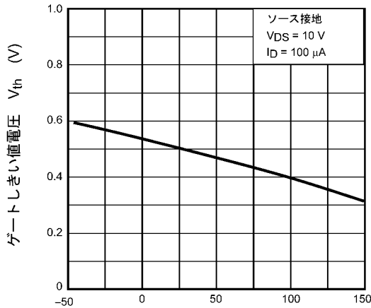
図 7.7 V_{th} - T_a
