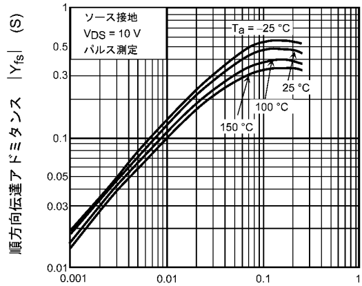
図 7.8 |Y_{fs}| - I_D
