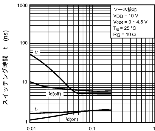
図 7.11 t - I_D
