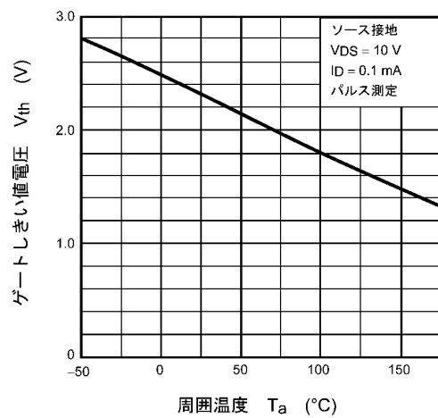
図 8.6 V_{th} - T_a
