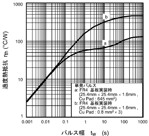
図 8.12 r_{th} - t_w
