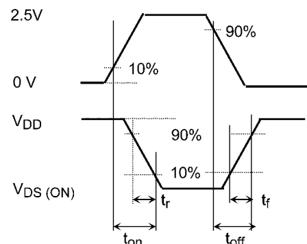
図 6.3.2 入力波形/出力波形
