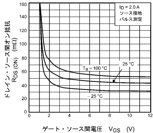
図 8.4 R_{DS(ON)} - V_{GS}
