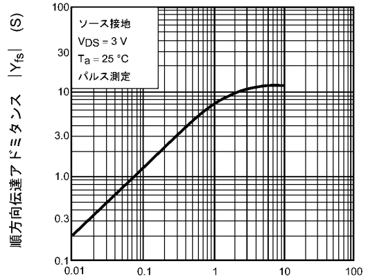
図 8.8 |Y_{fs}| - I_D
