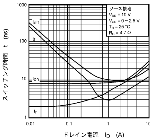
図 8.11 t - I_D
