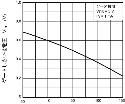
図 8.7 V_{th} - T_a
