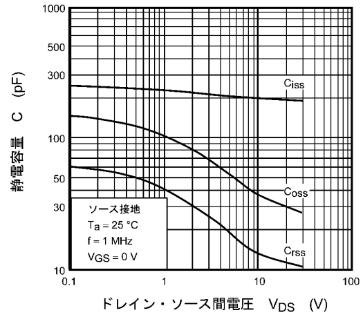
図 8.10 C - V_{DS}
