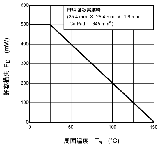
図 7.12 P_D - T_a
