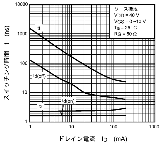
図 7.10 t - I_D
