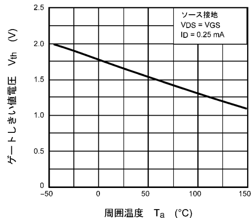
図 7.6 V_{th} - T_a
