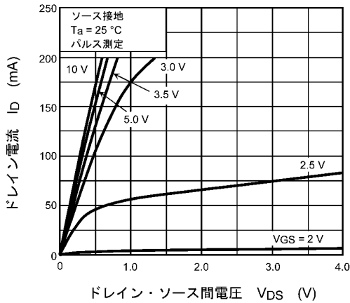
図 7.1 I_D - V_{DS}
