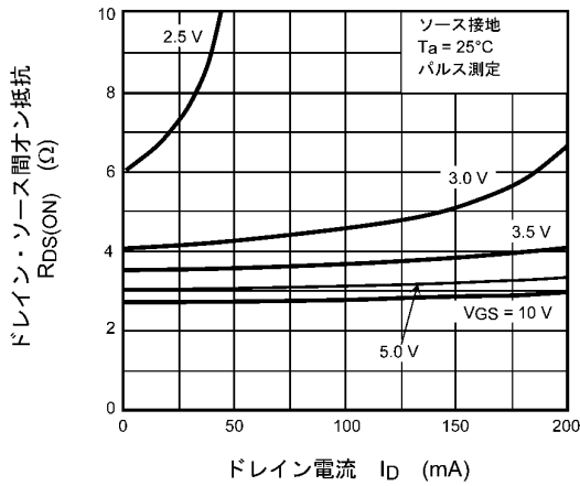
図 7.3 R_{DS(ON)} - I_D
