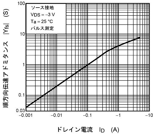
図 7.1.7 |Y_{fs}| - I_D
