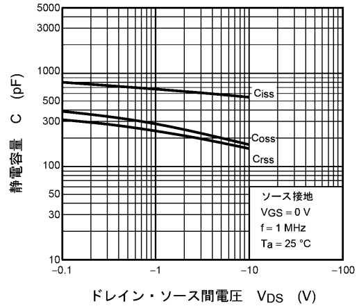
図 7.1.8 C - V_{DS}
