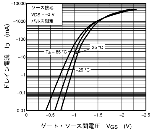
図 7.1.2 I_D - V_{GS}
