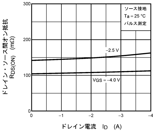
図 7.1.3 R_{DS(ON)} - I_D
