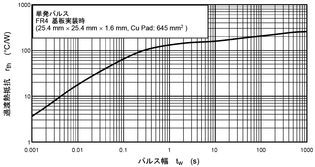
図 7.3.1 r_{th} - t_w (MOSFET部)
