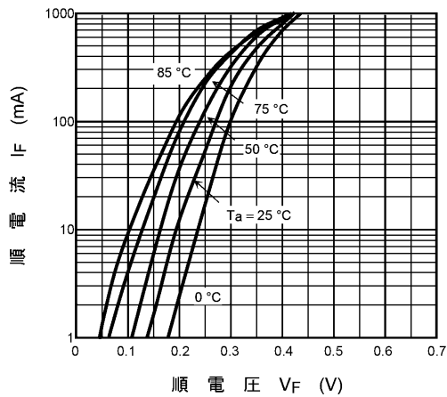
図 7.2.1 I_F - V_F
