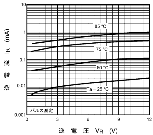
図 7.2.2 I_R - V_R
