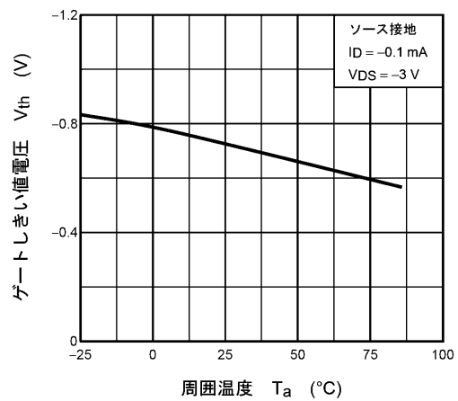
図 7.1.6 V_{th} - T_a
