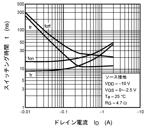
図 7.1.10 t - I_D
