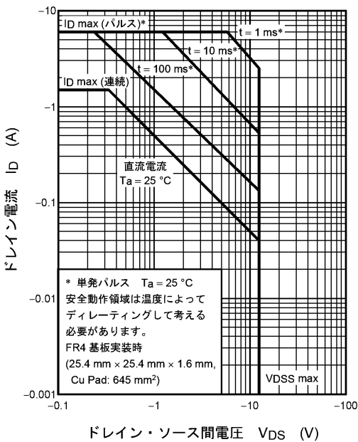
図 7.1.11 安全動作領域
