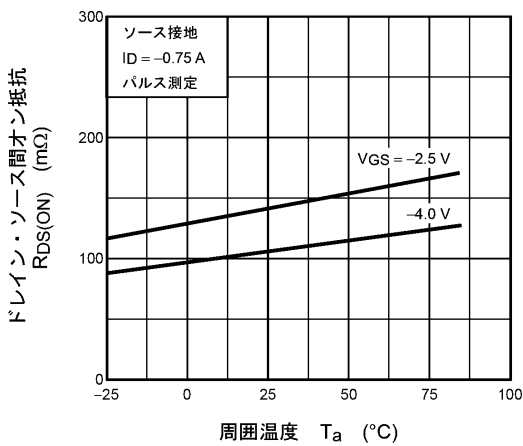
図 7.1.5 R_{DS(ON)} - T_a
