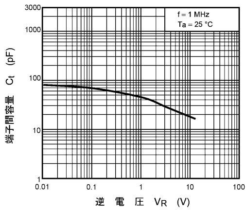
図 7.2.3 C_t - V_R
