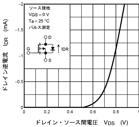
図 7.1.9 I_{DR} - V_{DS}
