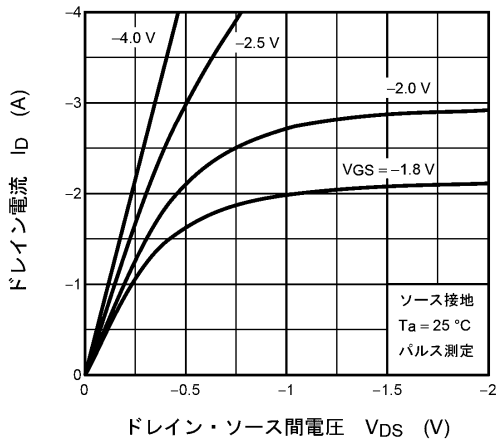
図 7.1.1 I_D - V_{DS}
