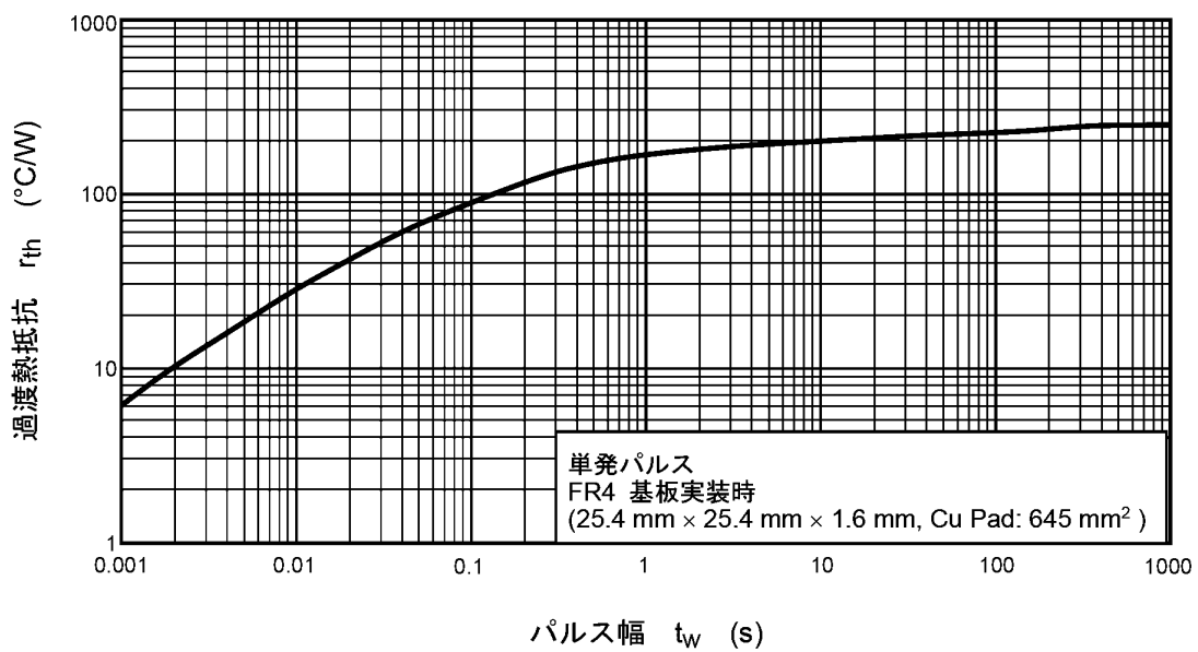
図 7.3.2 r_{th} - t_w (SBD部)
