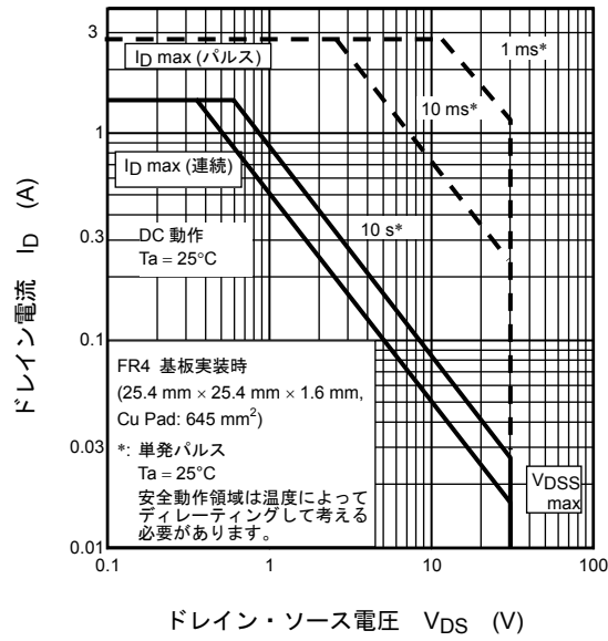
安全動作領域 (MOSFET 部)
