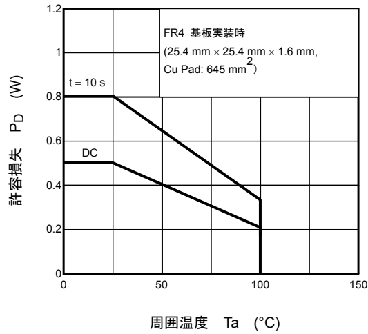
P_D - T_a (MOSFET 部)
