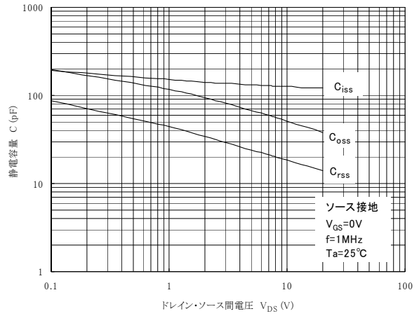
C - V_{DS} (MOSFET部)
