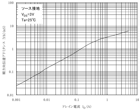
|Y_{fs}| - I_D (MOSFET部)
