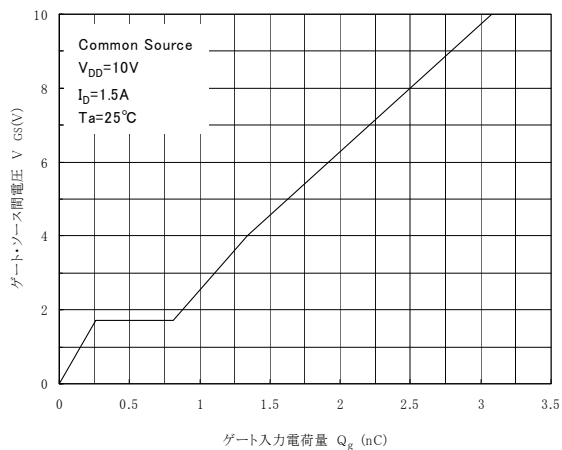
ダイナミック入力特性 (MOSFET)
