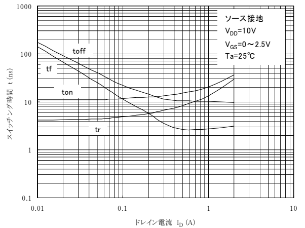
t - I_D (MOSFET部)
