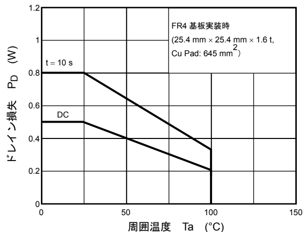
P_D - T_a (MOSFET部)
