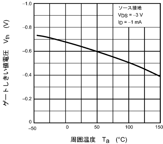
図 7.7 V_{th} - T_a
