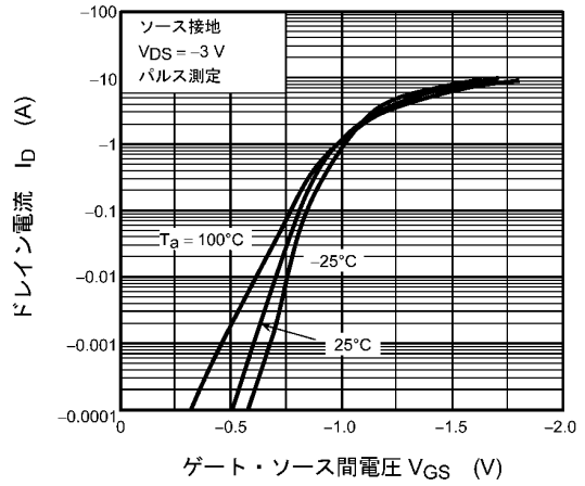
図 7.2 I_D - V_{GS}
