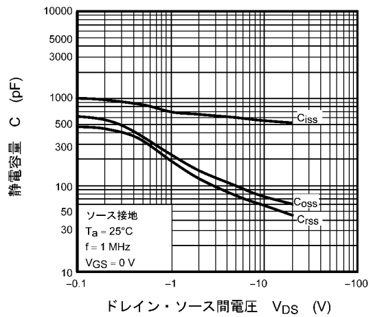
図 7.10 C - V_{DS}
