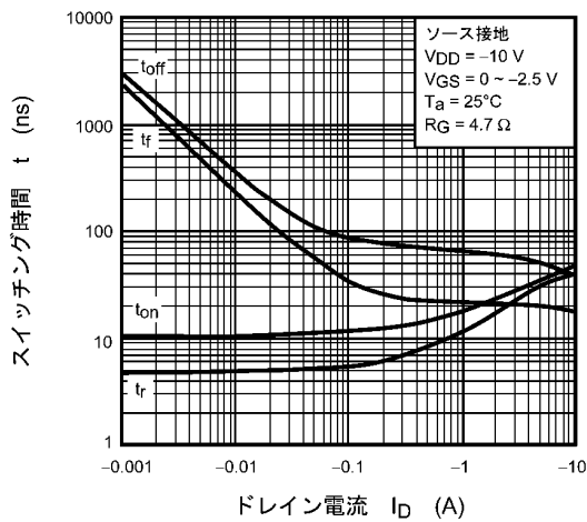
図 7.11 t - I_D
