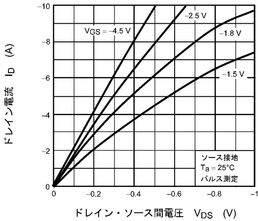
図 7.1 I_D - V_{DS}
