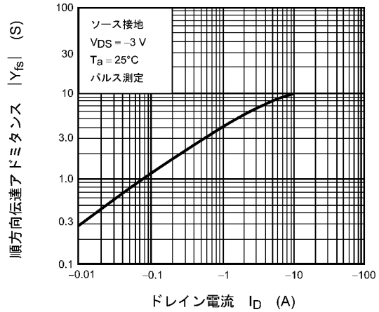
図 7.8 |Y_{fs}| - I_D
