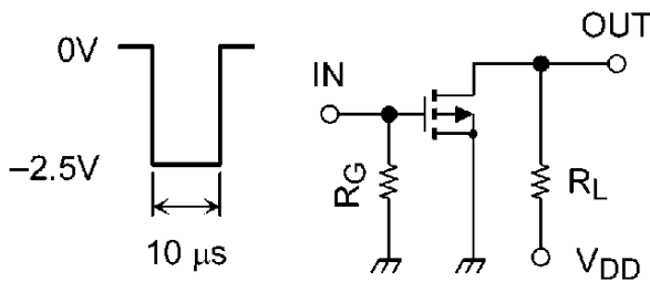
図 5.3.1 スwitching時間の測定回路
