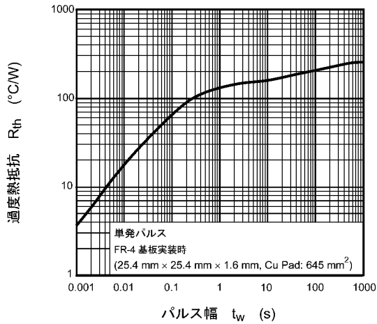
図 7.13 r_{th} - t_w
