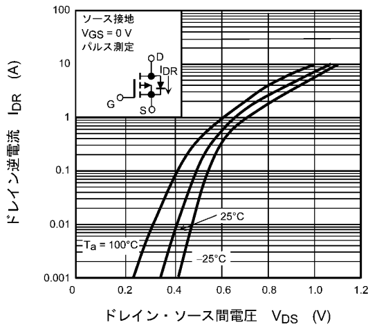
図 7.9 I_{DR} - V_{DS}
