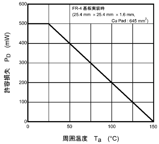
図 7.14 P_D - T_a
