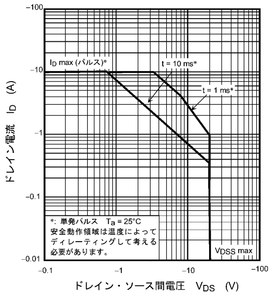
図 7.15 安全動作領域
