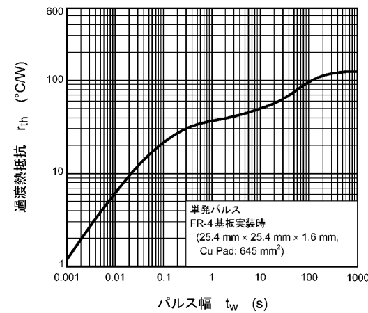
図 7.12 r_{th} - t_w
