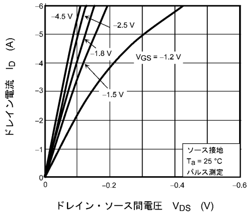
図 7.1 I_D - V_{DS}
