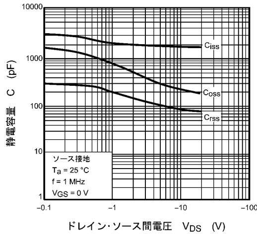
図 7.9 C - V_{DS}
