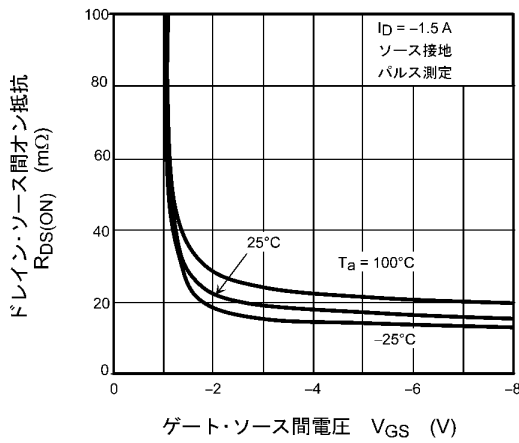
図 7.3 R_{DS(ON)} - V_{GS}
