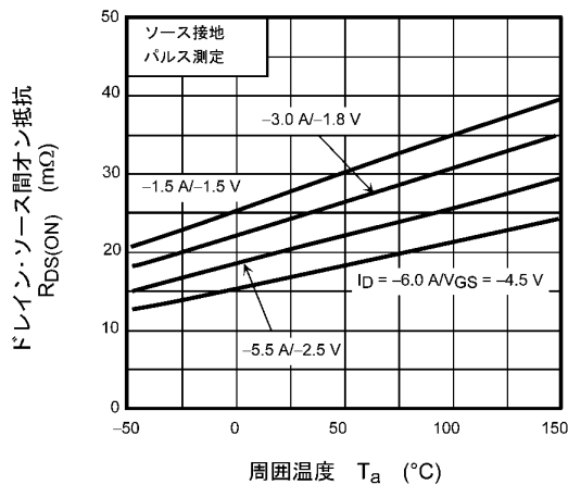
図 7.5 R_{DS(ON)} - T_a
