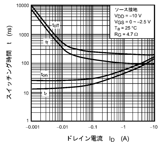
図 7.10 t - I_D
