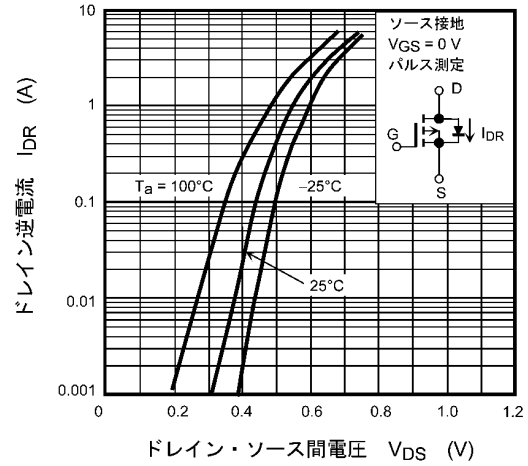
図 7.8 I_{Dr} - V_{DS}
