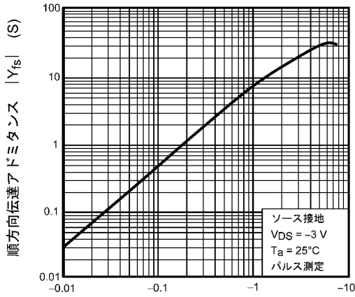
図 7.7 |Y_{fs}| - I_D
