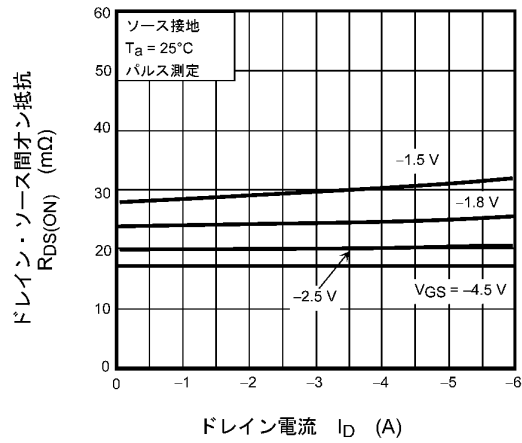
図 7.4 R_{DS(ON)} - I_D
