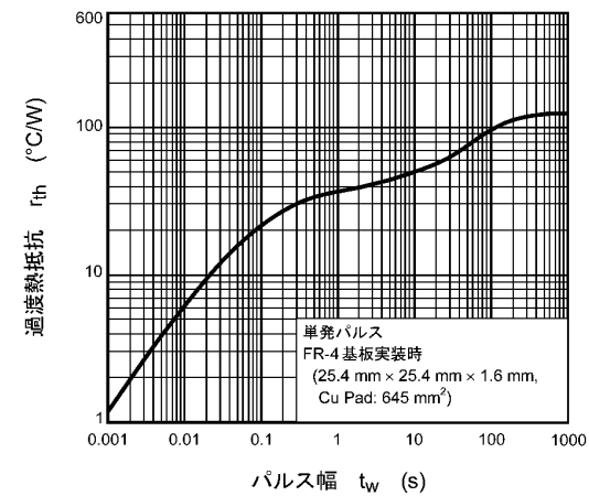
図 7.12 r_{th} - t_w
