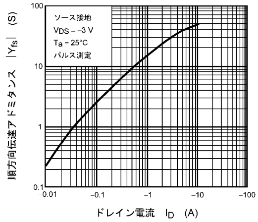
図 8.8 |Y_{fs}| - I_D
