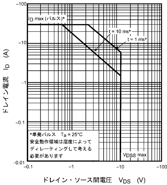
図 8.15 安全動作領域
