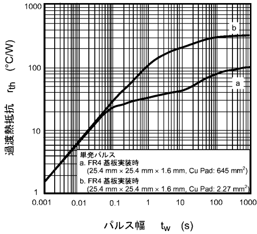
図 8.13 r_{th} - t_w
