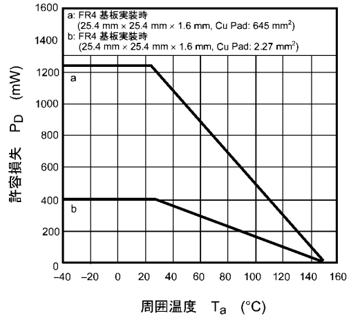
図 8.14 P_D - T_a
