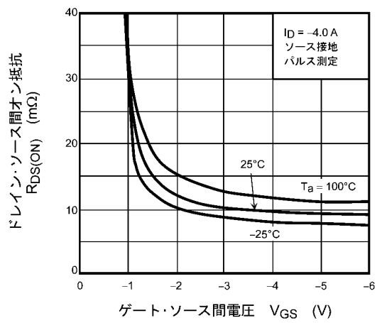
図 8.4 R_{DS(ON)} - V_{GS}
