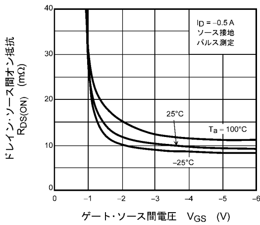
図 8.3 R_{DS(ON)} - V_{GS}
