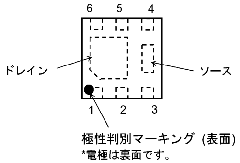
図 6.2 ピン配置(Top View)
