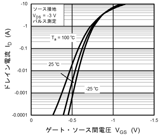
図 7.2 I_D - V_{GS}
