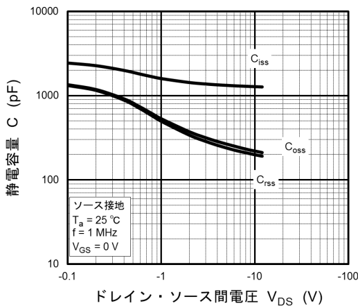
図 7.9 C - V_{DS}
