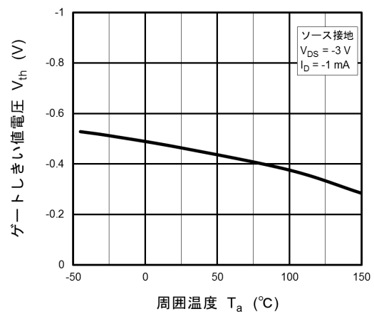
図 7.6 V_{th} - T_a
