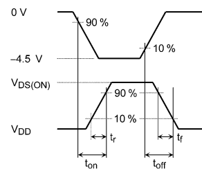
図 5.3.2 入力波形/出力波形
