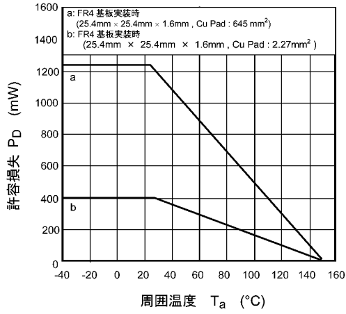
図 7.13 P_D - T_a
