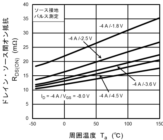
図 7.5 R_{DS(ON)} - T_a
