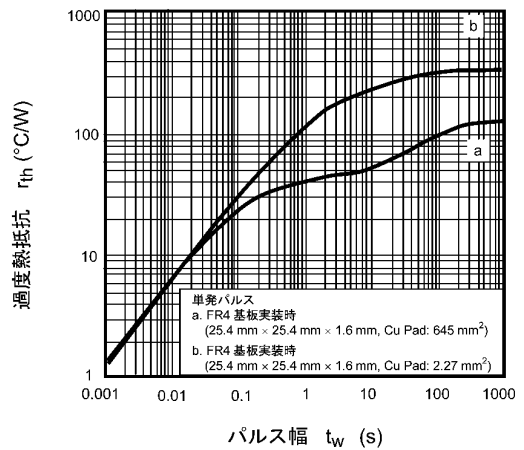
図 7.12 r_{th} - t_w
