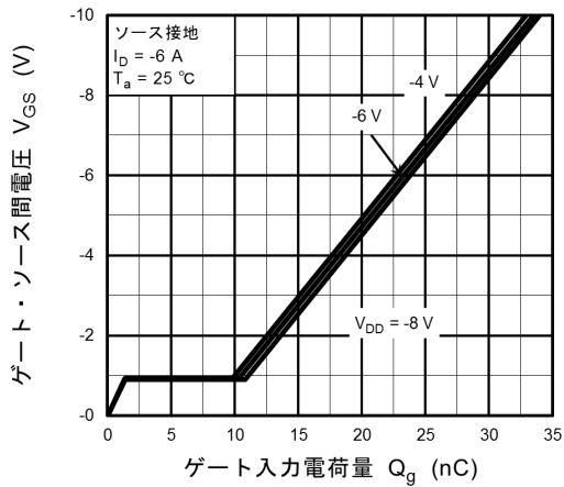
図 7.11 ダイナミック入力特性
