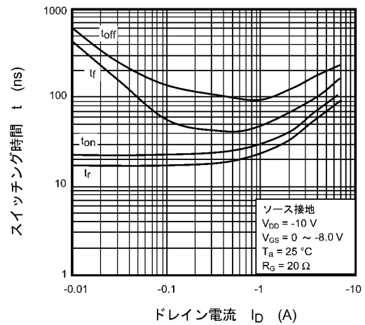
図 7.10 t - I_D
