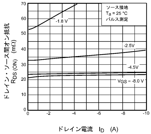
図 7.4 R_{DS(ON)} - I_D
