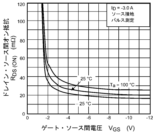
図 7.3 R_{DS(ON)} - V_{GS}
