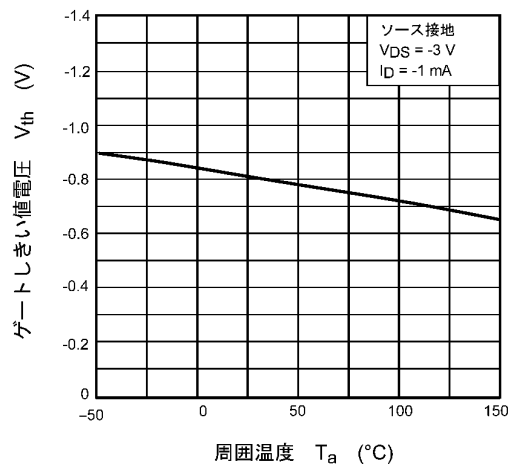
図 7.6 V_{th} - T_a
