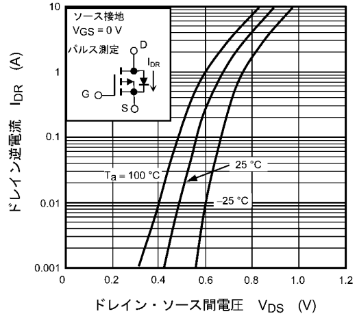
図 7.8 I_{DR} - V_{DS}
