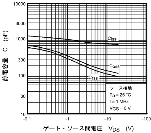
図 7.9 C - V_{DS}
