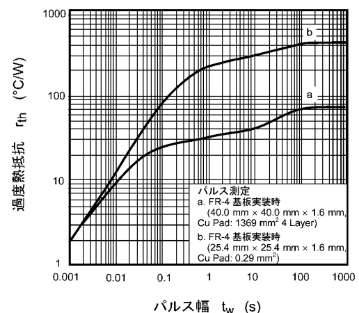
図 7.12 r_{th} - t_w
