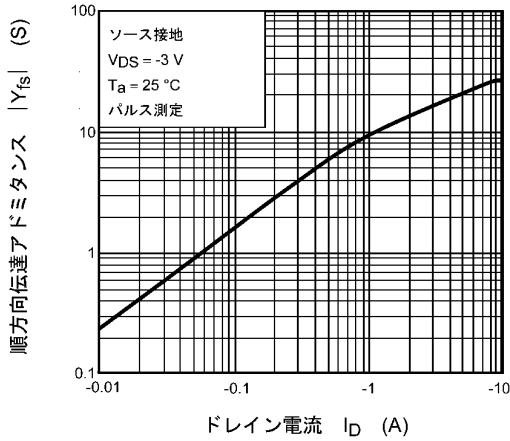
図 7.7 |Y_{fs}| - I_D
