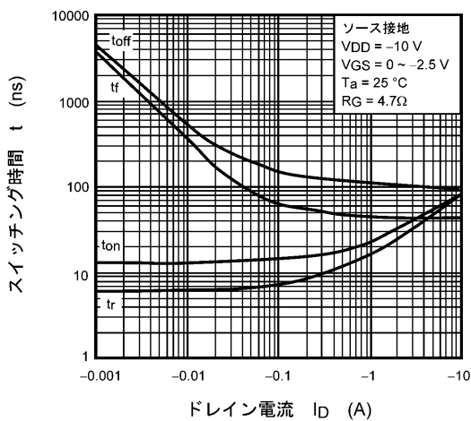
図 7.11 t - I_D
