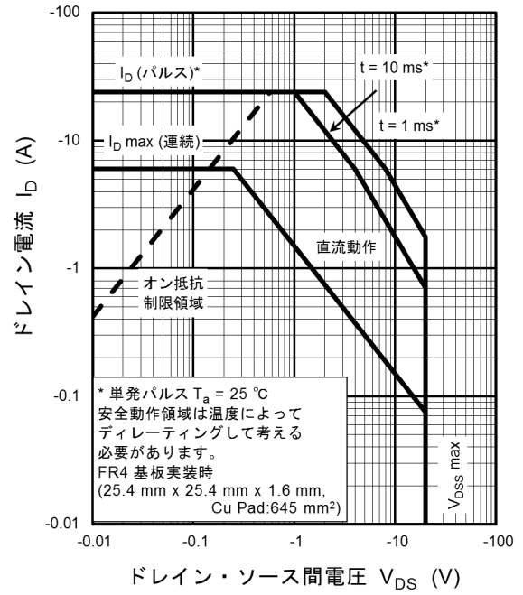
図 7.14 安全動作領域
