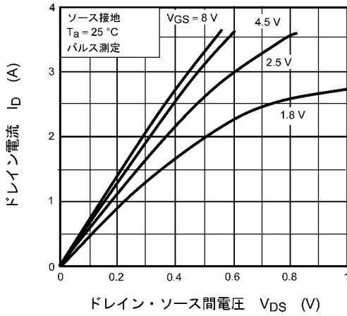
図 7.1 I_D - V_{DS}
