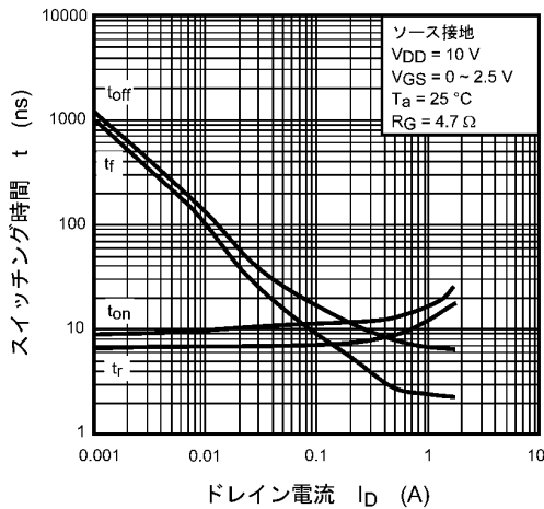
図 7.11 t - I_D
