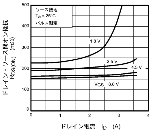
図 7.5 R_{DS(ON)} - I_D
