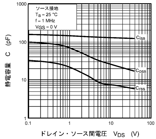
図 7.10 C - V_{DS}
