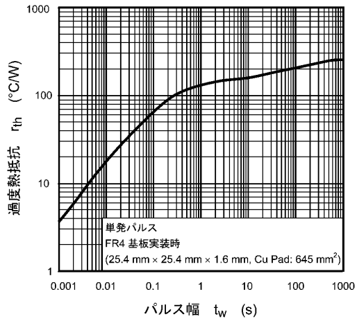
図 7.13 r_{th} - t_w
