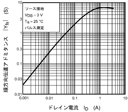
図 7.8 |Y_{fs}| - I_D
